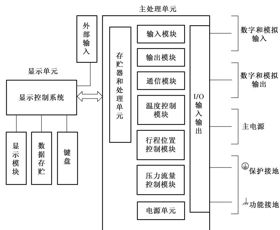
图 B.1 塑料机械计算机控制系统框图
